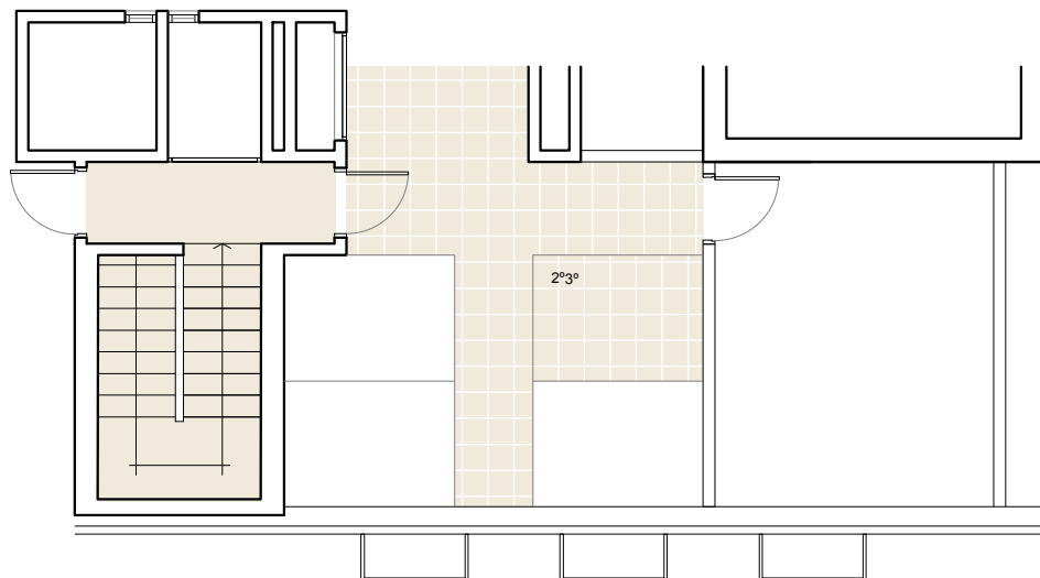
PLANTA COBERTA
