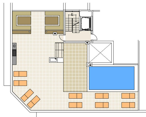
PLANTA PRIMERA COBERTA 1/200
